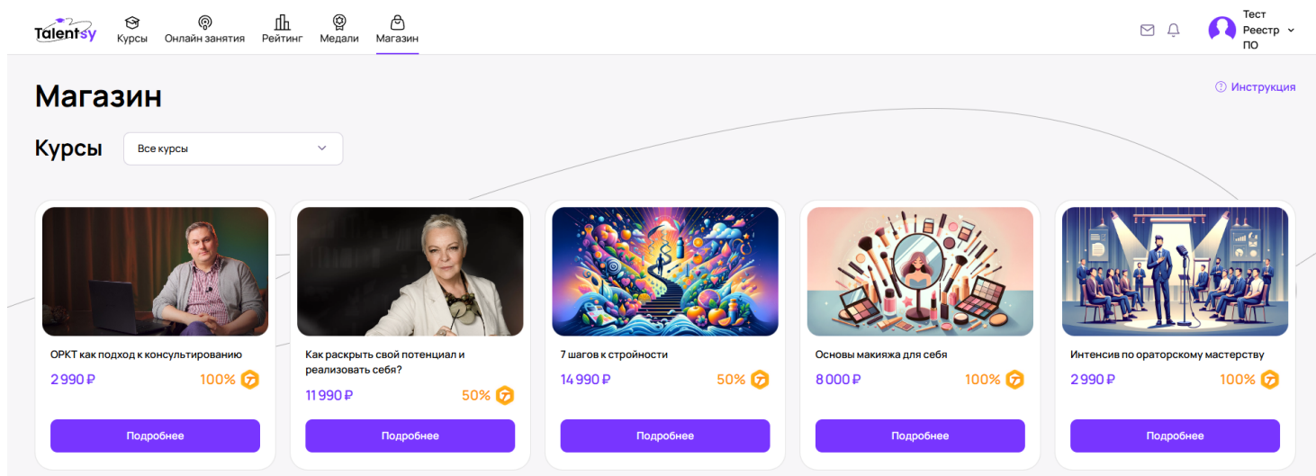
Рисунок 8 – Окно магазин.
