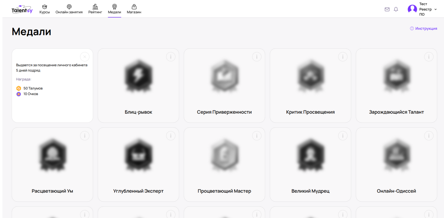
Рисунок 7 – Окно медали.
