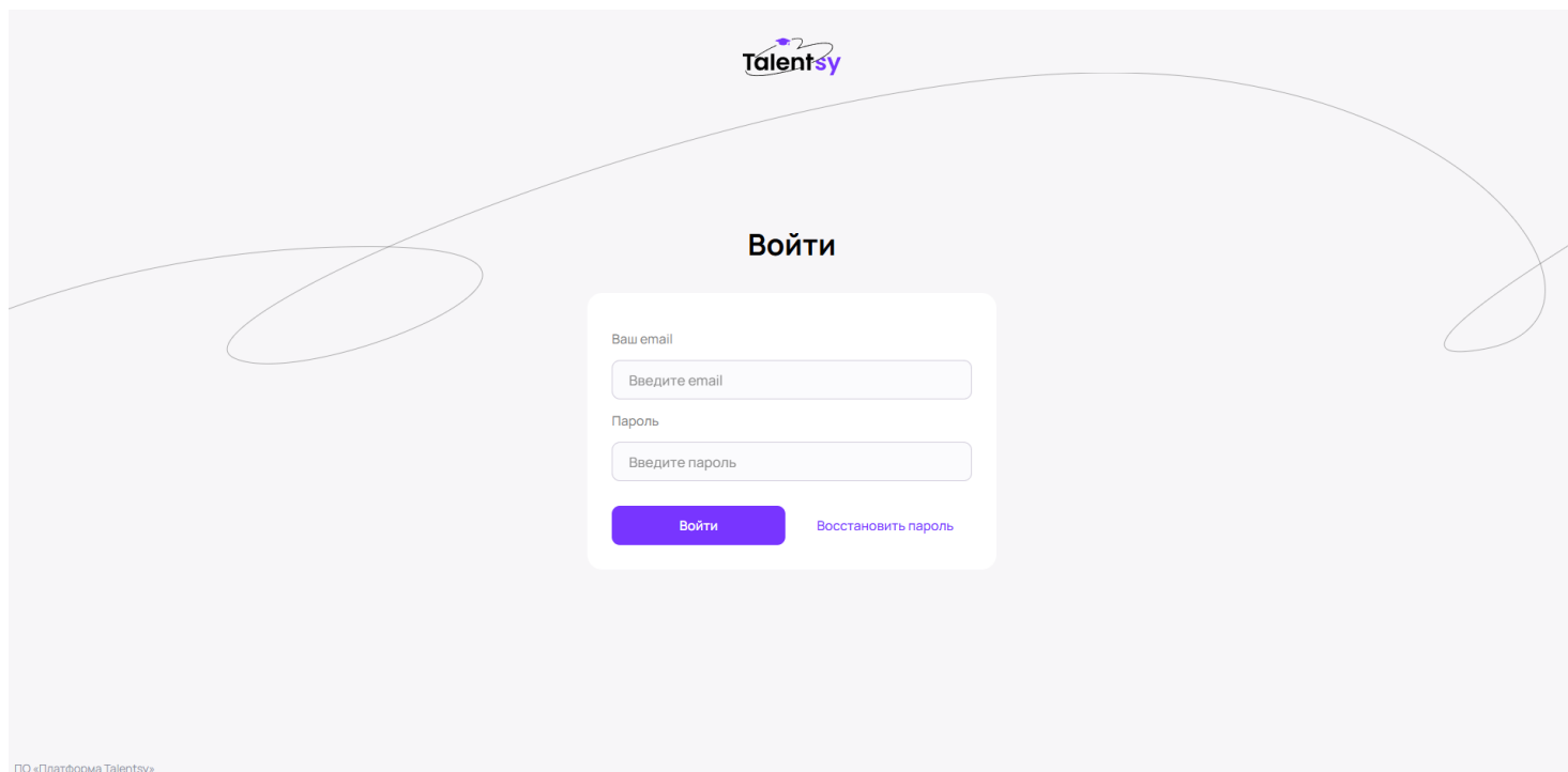
Рисунок 1 – Окно авторизации.
