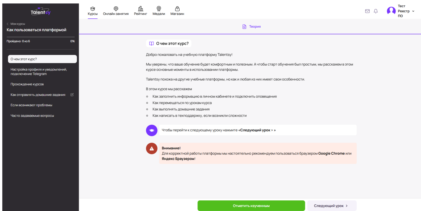
Рисунок 4 – Окно курса.
