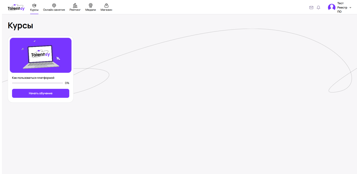
Рисунок 3 – Окно курсы.
