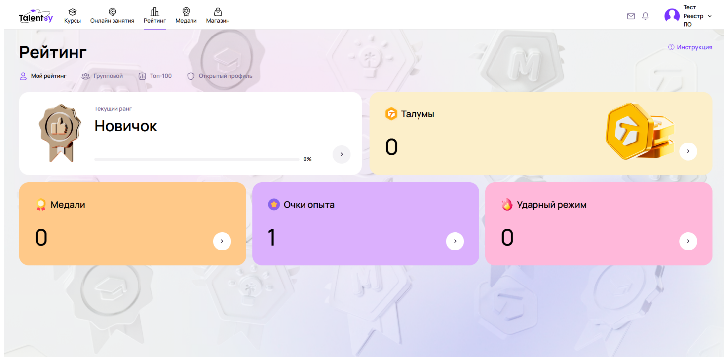
Рисунок 6 – рейтинг.
